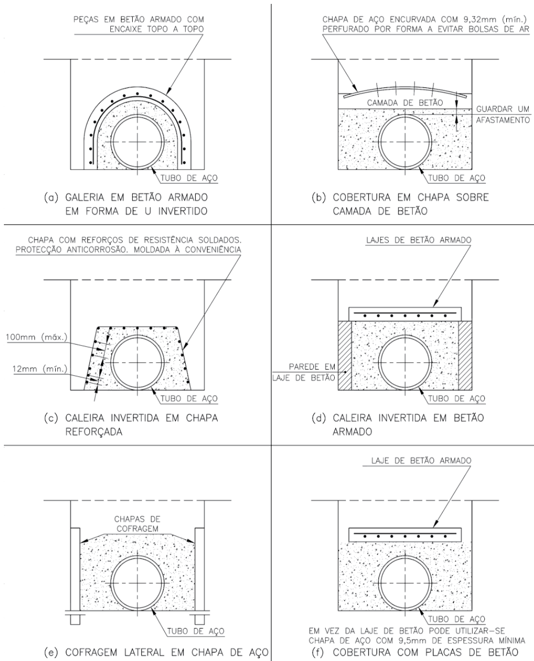
Fig. 2 — Medidas de segurança suplementares
