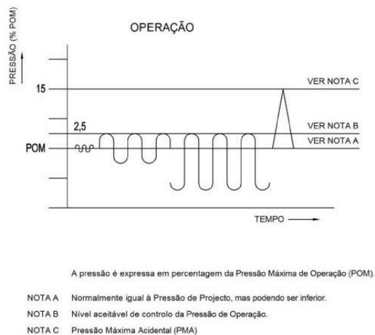
Fig. 1 — Guia para sistemas de limitação de pressão
